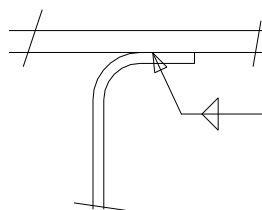
Figura 65.2.3.b. Detalle a evitar para la soldadura del perno a la placa base
