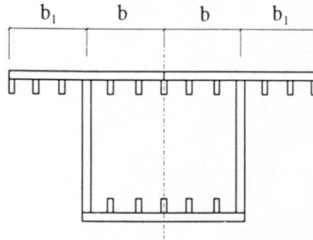
Figura 21.4. Anchuras eficaces en alas rigidizadas.
