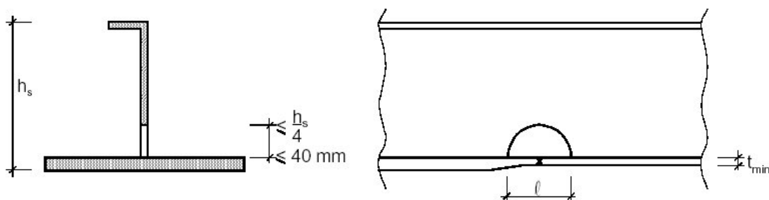
Figura A7.2.4.a. Agujeros en rigidizadores longitudinales
