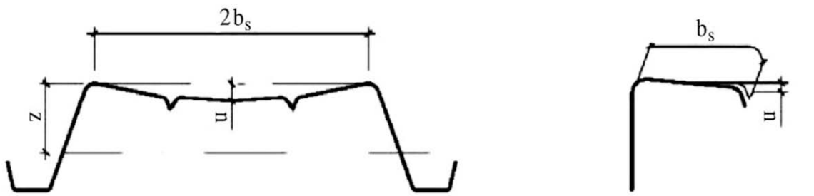
Figura 73.7. Combadura de alas (u)
