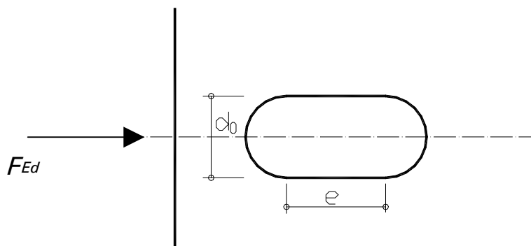
Figura 58.3. Agujeros rasgados
