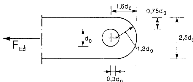
Figura 58.9.b
